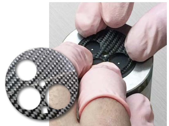
La pièce en carbone est appliquée sur l'adhésif double face
