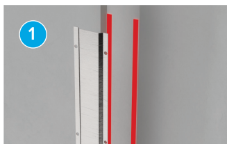
1 Befestigung von Schienen und Versteifungsstreben tesa® ACX plus 78xx Serie
