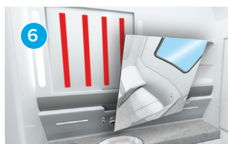
6 Spiegelverklebung → tesa® 4952
