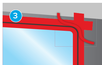
Masquage pour processus d'étanchéité → tesa® 4174
