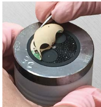
Schutzpapier wird von doppel-seitigem Klebeband abgezogen
